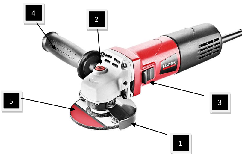
Фото 1 Загальний вид машини AG 780
